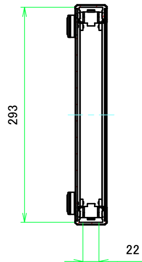
A-A (1:5)
